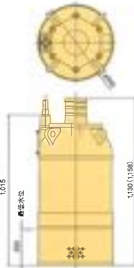
U-4306D・4308 ※ ( ) 内寸法はU-4308
